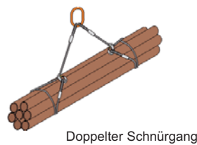
Doppelter Schnürgang
